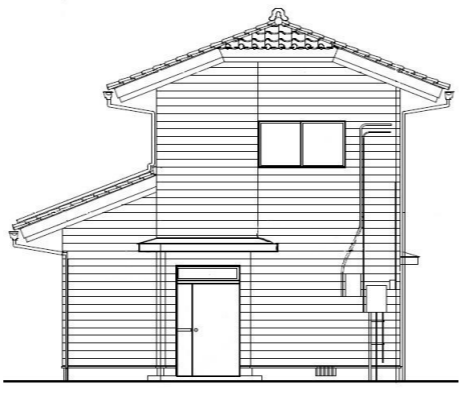
東立面図
