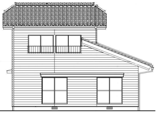
南立面図
