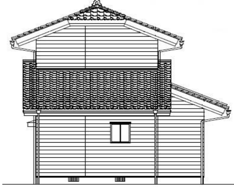
西立面図
