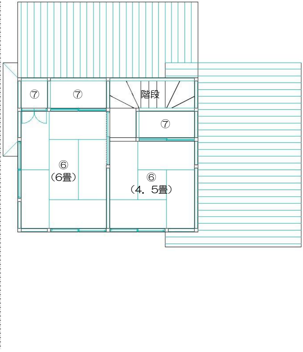
2階平面図
