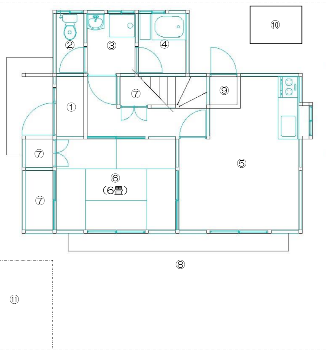
1階平面図
