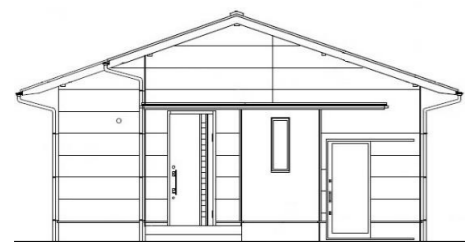
東立面
