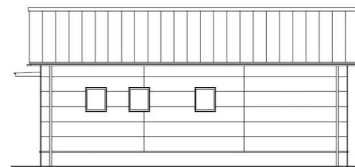
北立面
