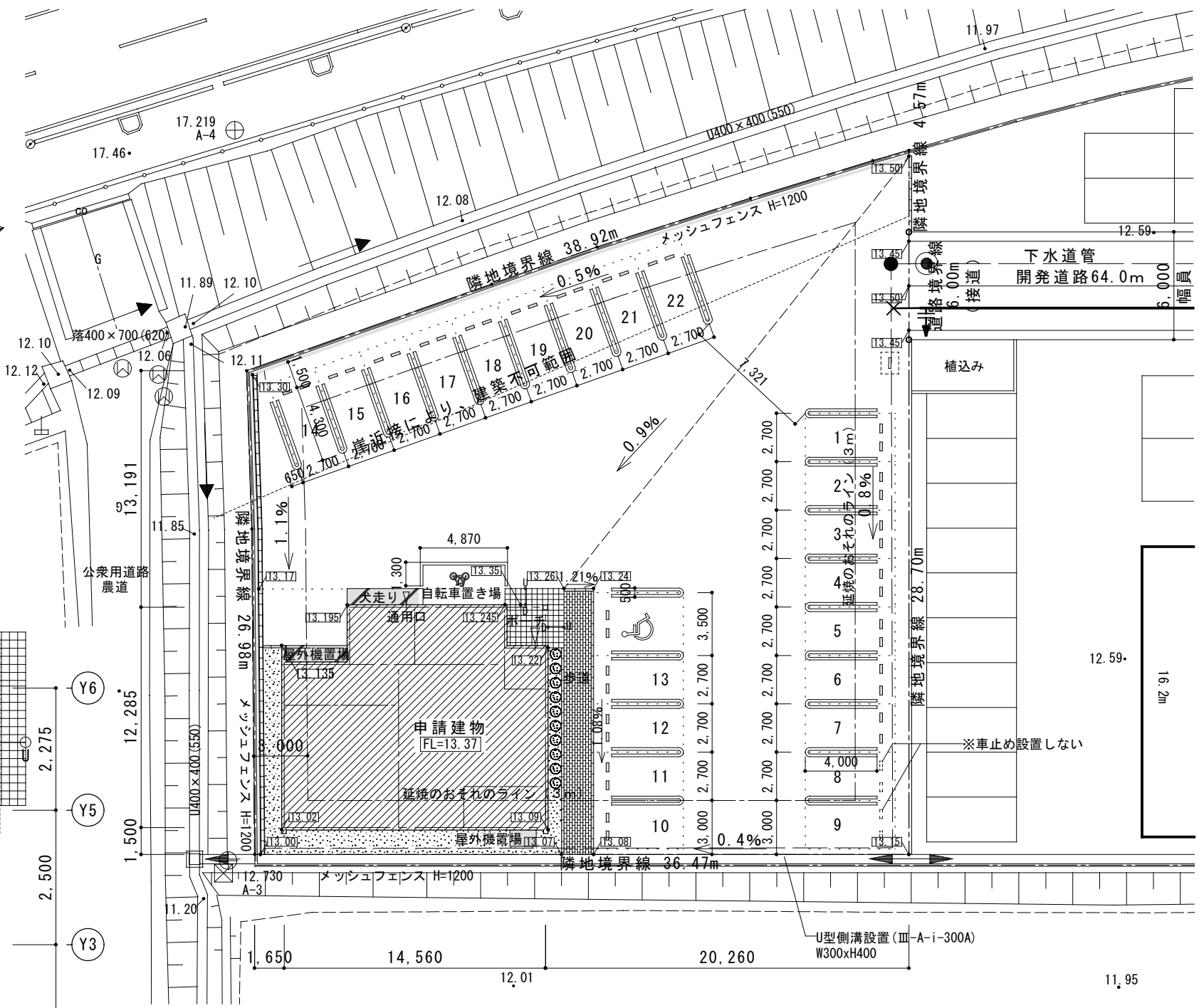
配置図
