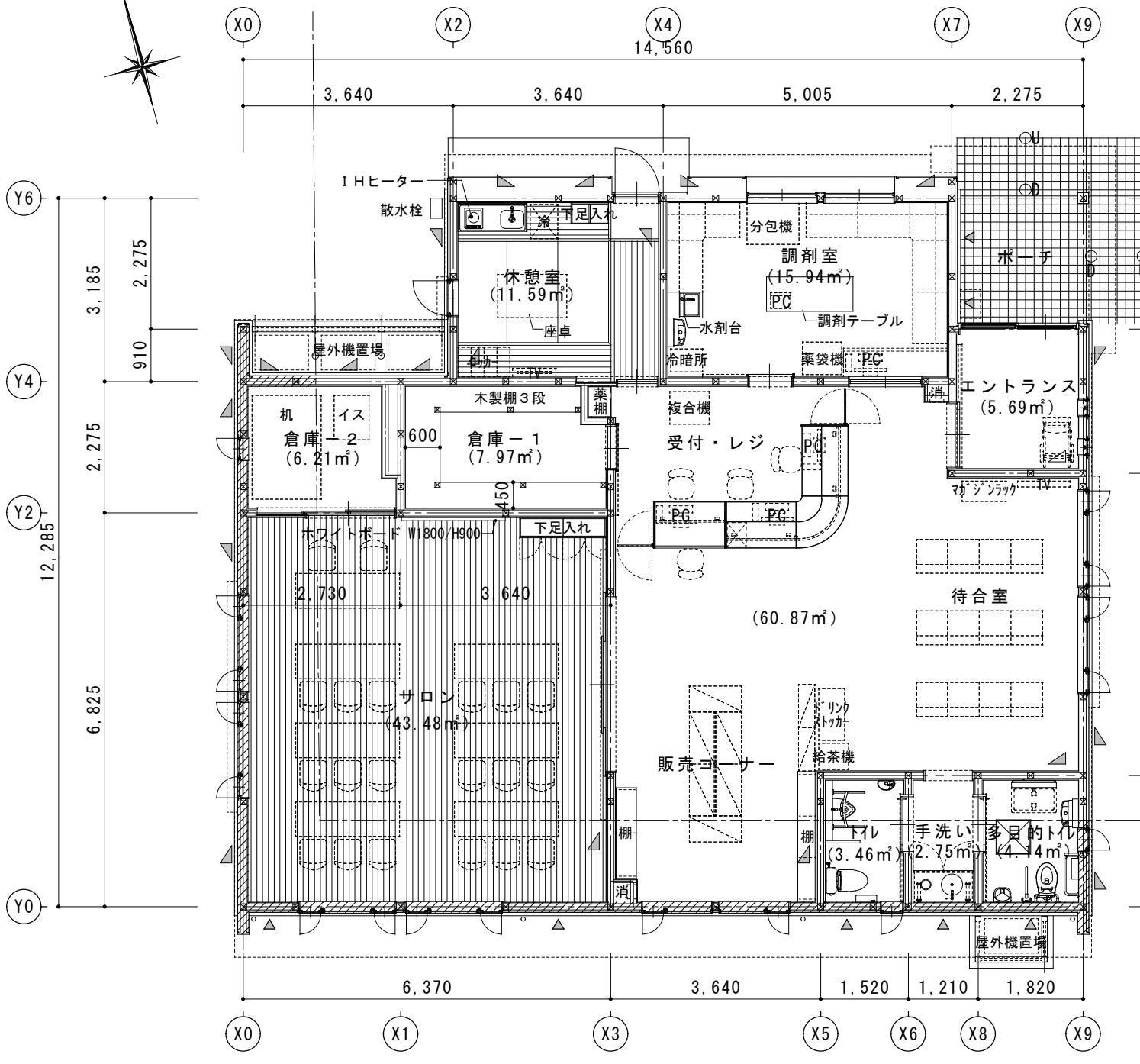
平面図
