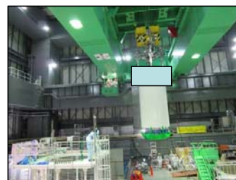
⑤使用済燃料プールキャスク着水
